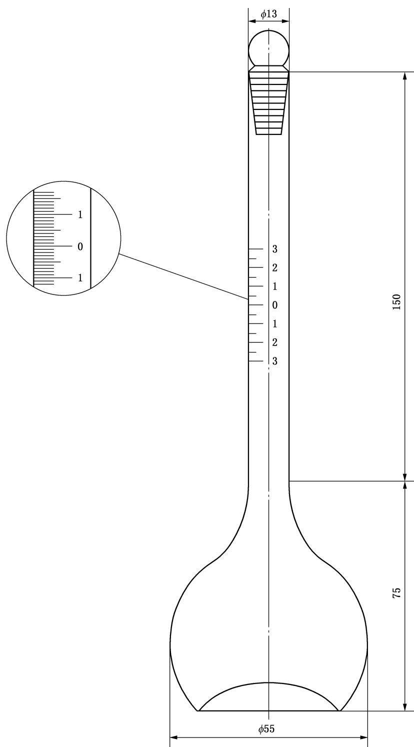
图 B. 1 稳定性试验用细颈容量瓶
