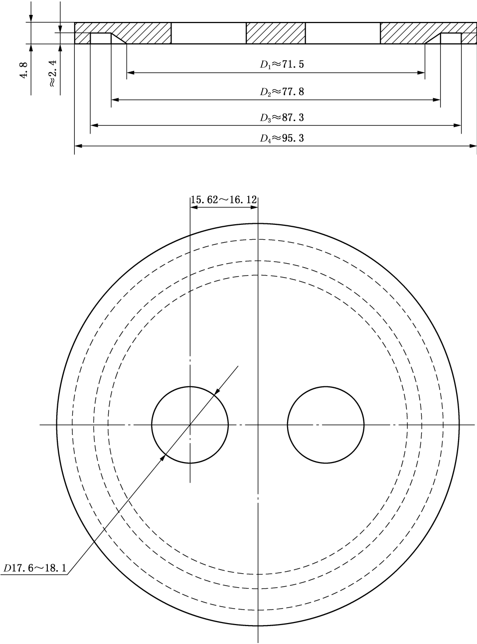
图 B. 2 防腐蚀试验用烧杯盖
