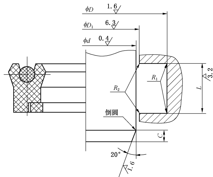
图 7 活塞杆复合密封沟槽型式
