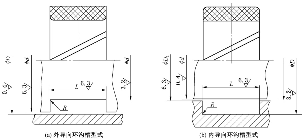
图 9 导向环沟槽型式
