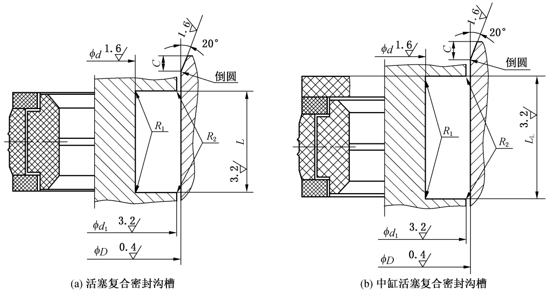
图 6 带挡圈的活塞复合密封沟槽型式
