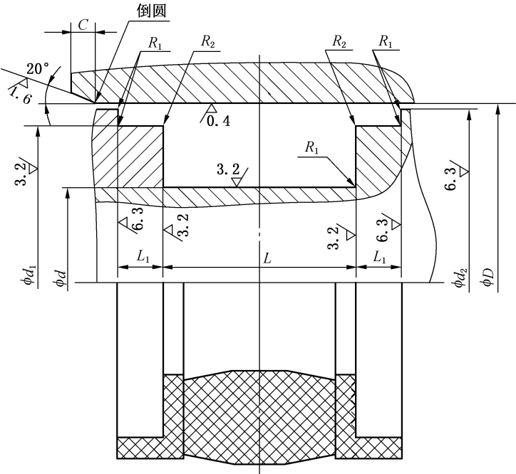
图 3 鼓形静密封沟槽型式
