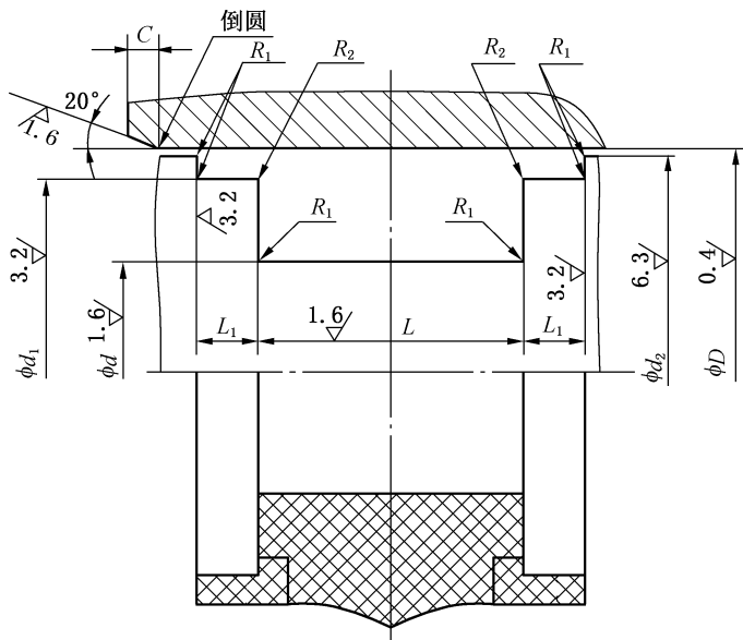
图 2 山形密封圈密封沟槽型式
