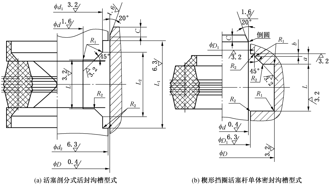
图 5 带楔形挡环的单体密封圈密封沟槽型式
