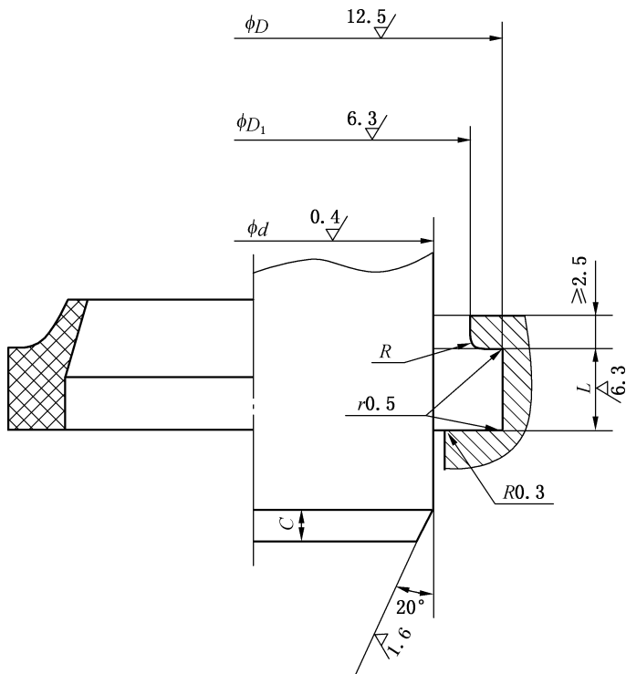
图 10 防尘圈沟槽型式
