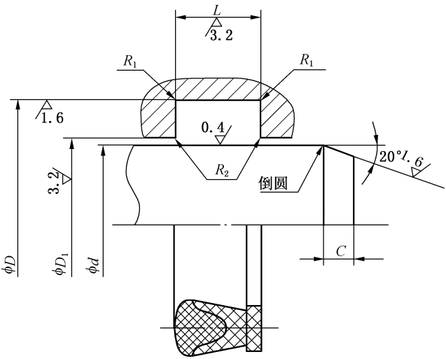
图 4 内蕾形密封圈沟槽型式
