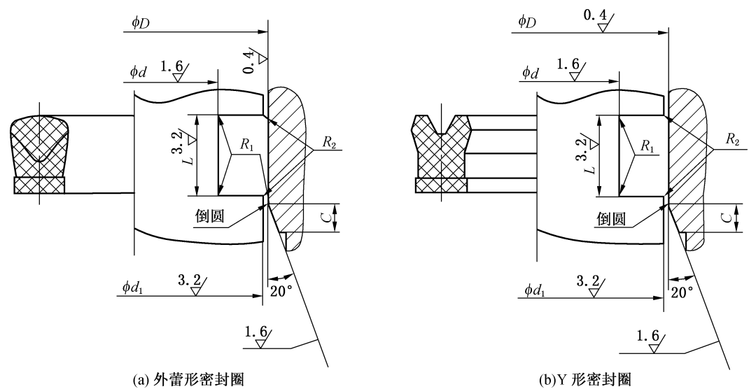
图 1 外蕾形密封圈和 Y 形密封圈沟槽型式
