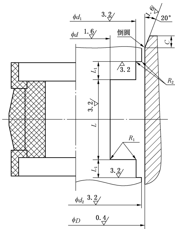
图 8 带 L 形挡圈的复合密封沟槽型式
