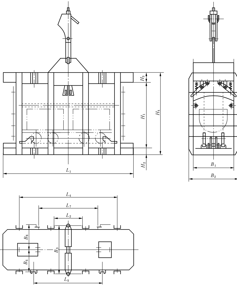
图 5 1t 矿车一层二车钢轨罐道罐笼
