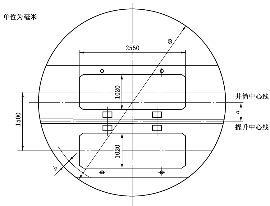
图 C.4 1t 矿车一层一车钢丝绳罐道罐笼
