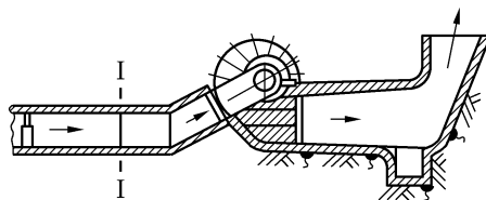
图3 离心式通风机测压断面位置图
