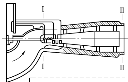
图2 轴流式通风机测压断面位置图
