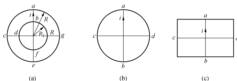
图 1 静压测点安设位置示意图
