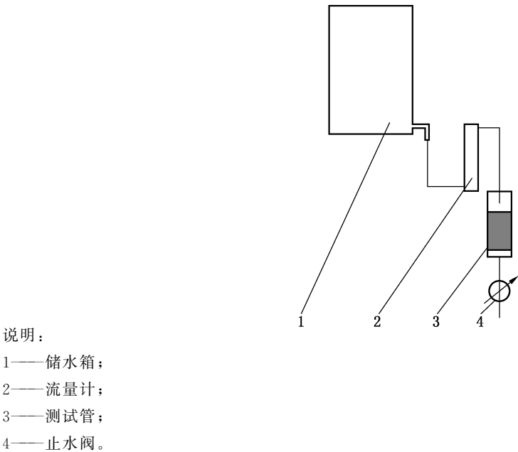
图 1 活性半脱氯值的试验装置
