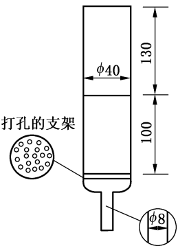
图 2 测试管
