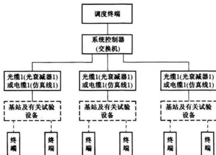
图3 星形系统总线型系统设备连接
