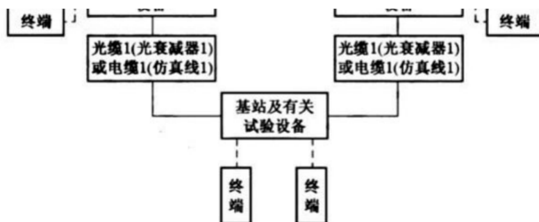
图2 环形系统设备连接
