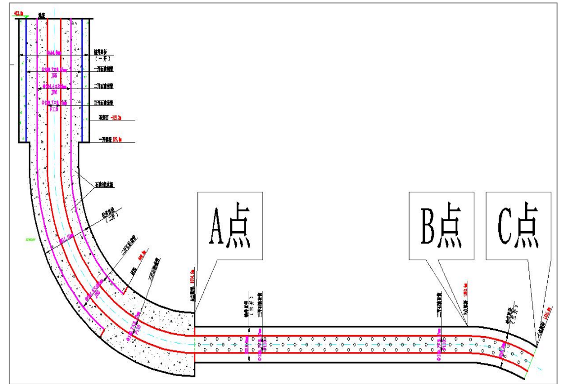
L型卸压井结构图
