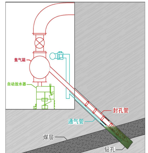
下向孔吹水示装置示意图
